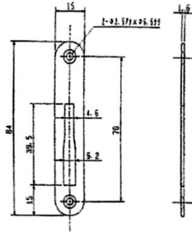
ストライクプレート寸法図
