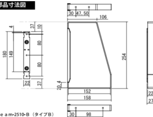
部品寸法図
