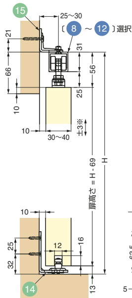
壁付仕様 使用例
