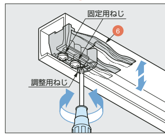
上図のようにねじを回してキャッチ力を調整できます。
