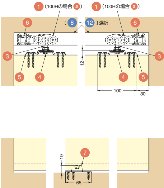
ハンガーパーツ⑤取付穴位置
