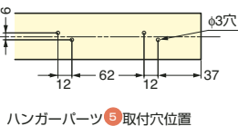
ハンガーパーツ⑤取付穴位置
