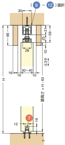
天付仕様 使用例
